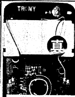
真 fx-991EX內部 太陽能、電池雙電源供應品質佳，內部電路板線路優良
