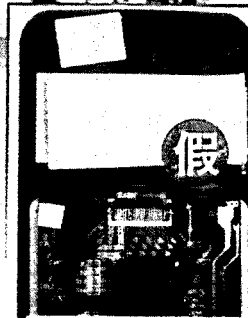
仿 fx-991EX內部 假太陽板不供電，電池規格可能不符政府標準，電路板質差線路不良
